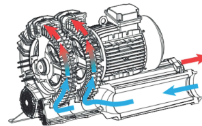
TS twin impeller single stage doppia girante singolo stadio doble impulsor mono etapa
